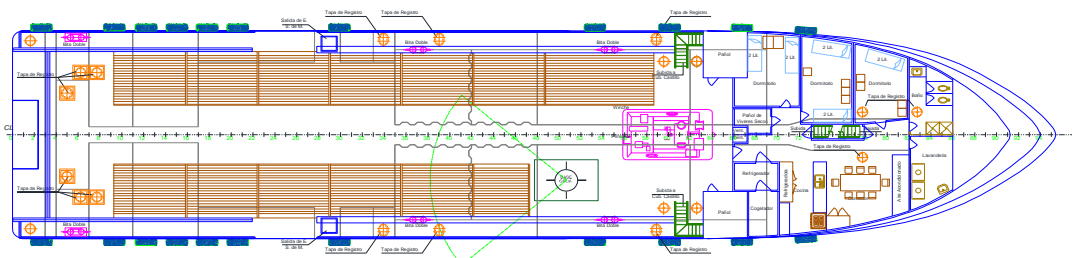
VISTA DE PLANTA "CUBIERTA PRINCIPAL"
