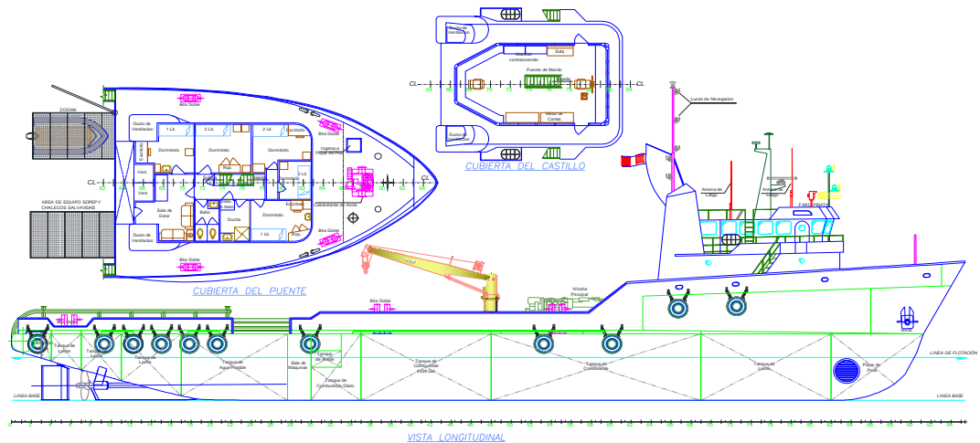
VISTA LONGITUDINAL
